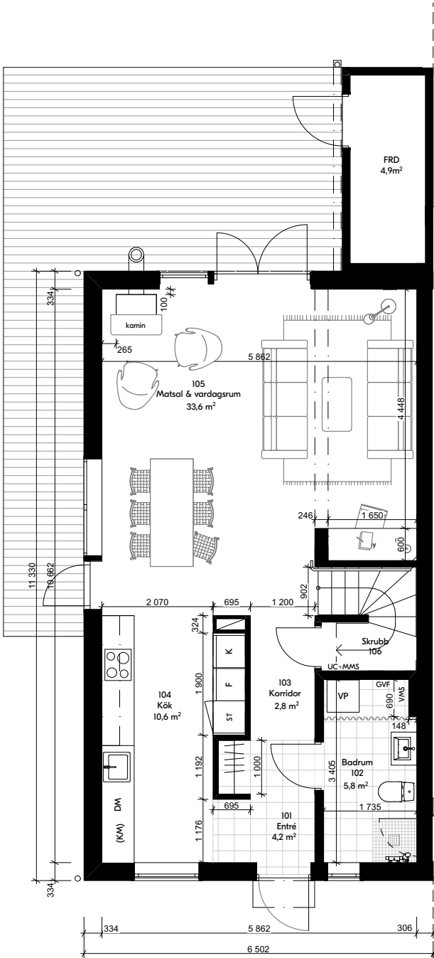
Entréplan
