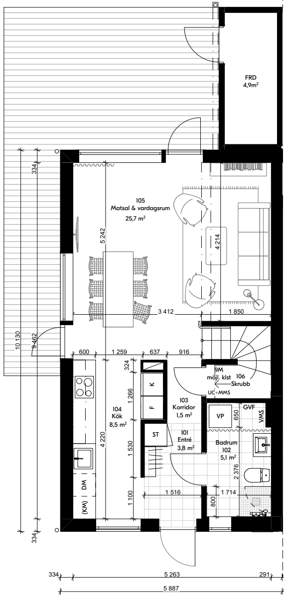
Entréplan
