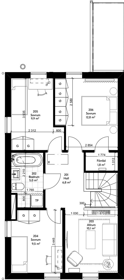
Övre plan
