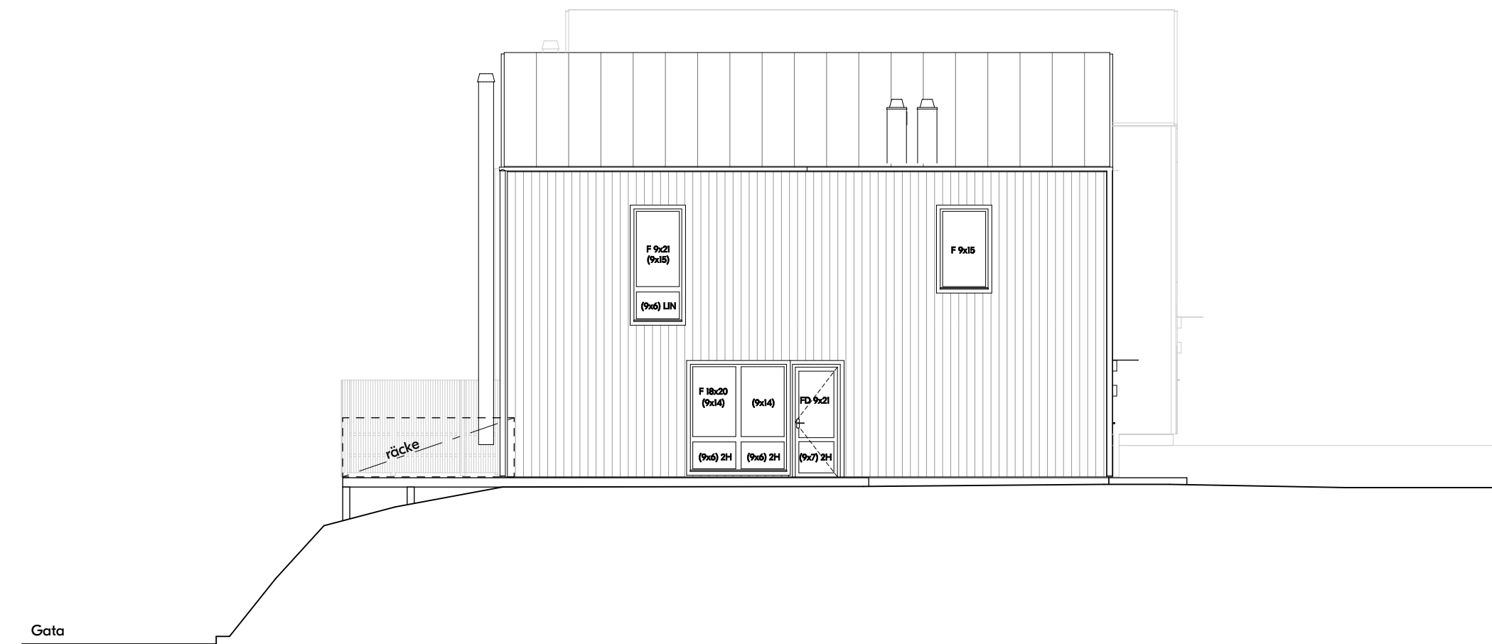
Gavel vänster
