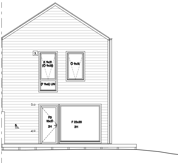
Baksida
