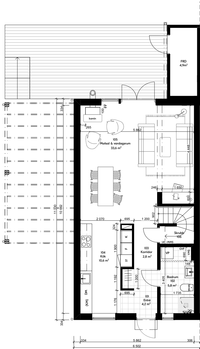
Entréplan
