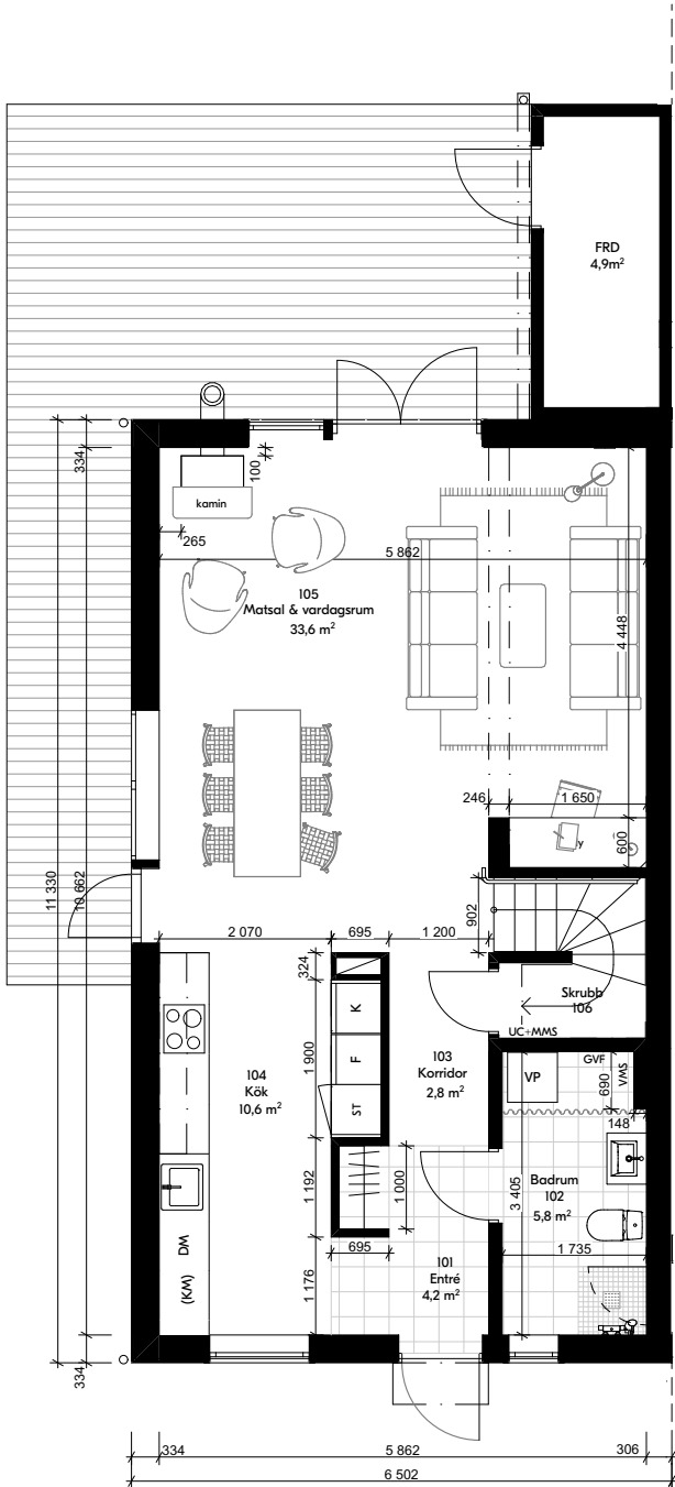
Entréplan
