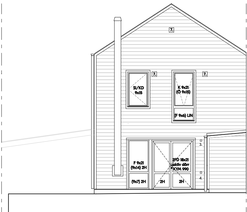
Baksida
