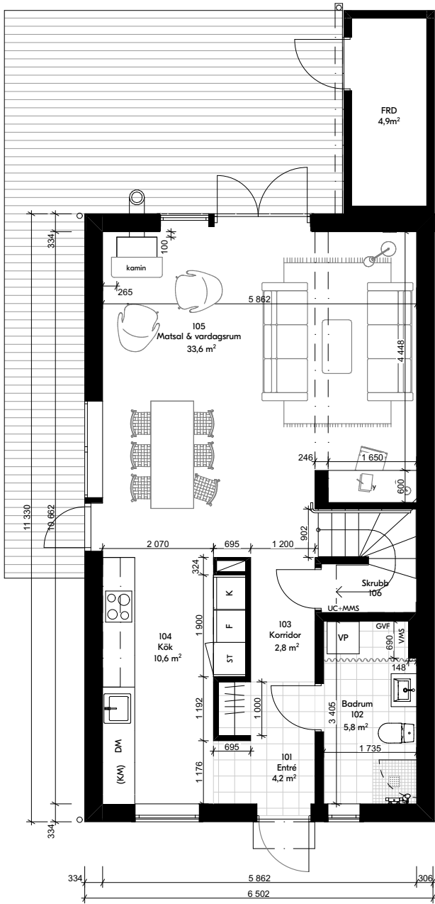
Entréplan
