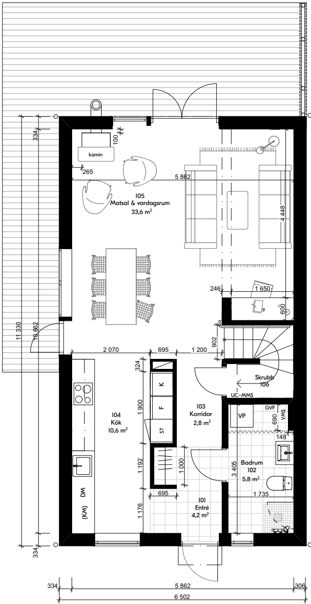
Entréplan
