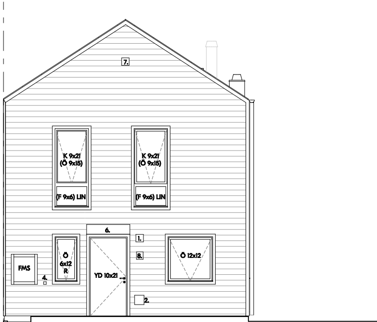
Framsida
