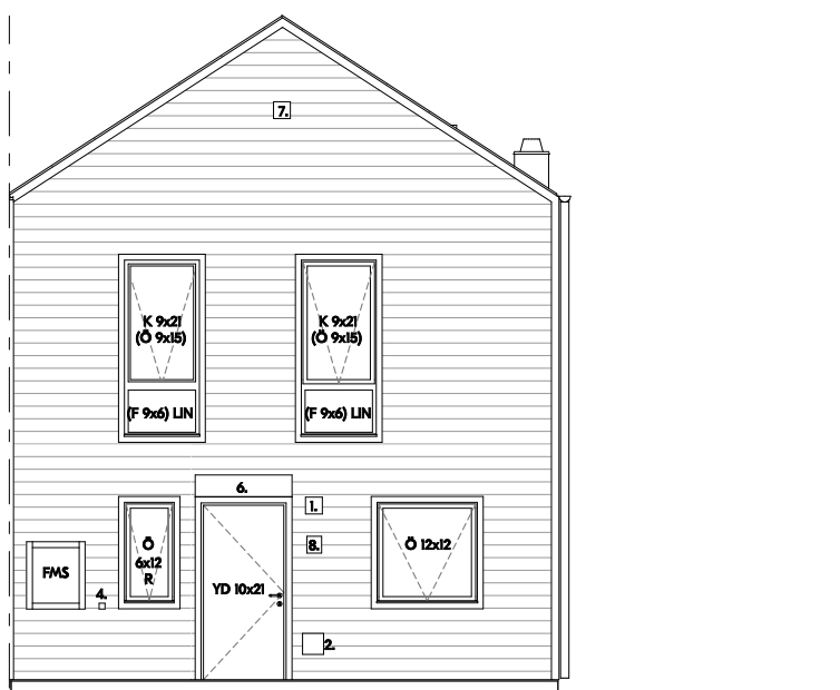
Framsida
