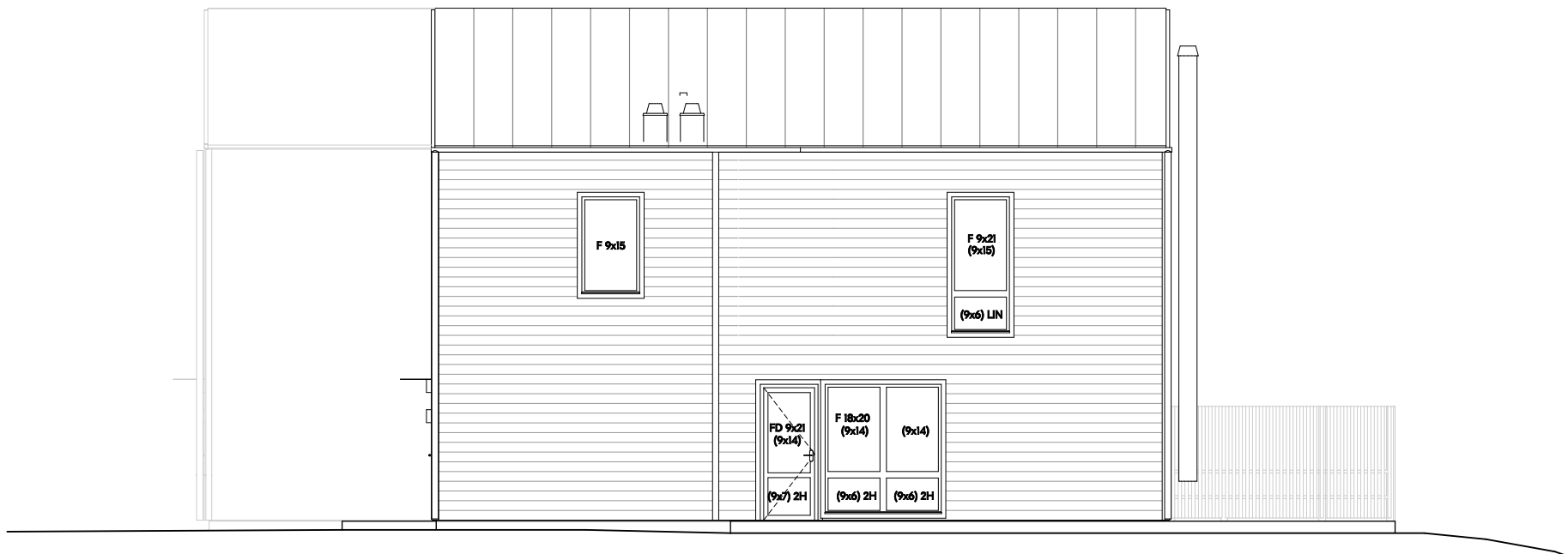
Gavel höger
