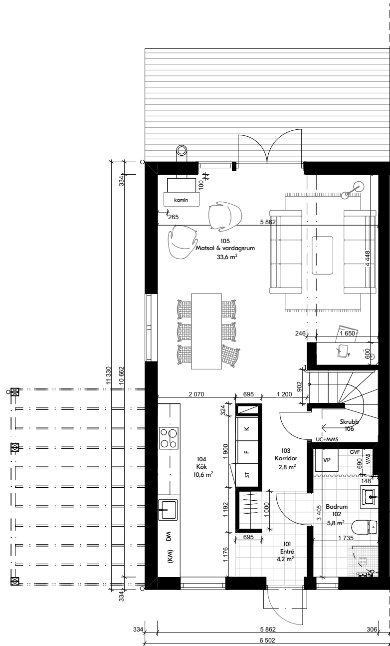
Entréplan
