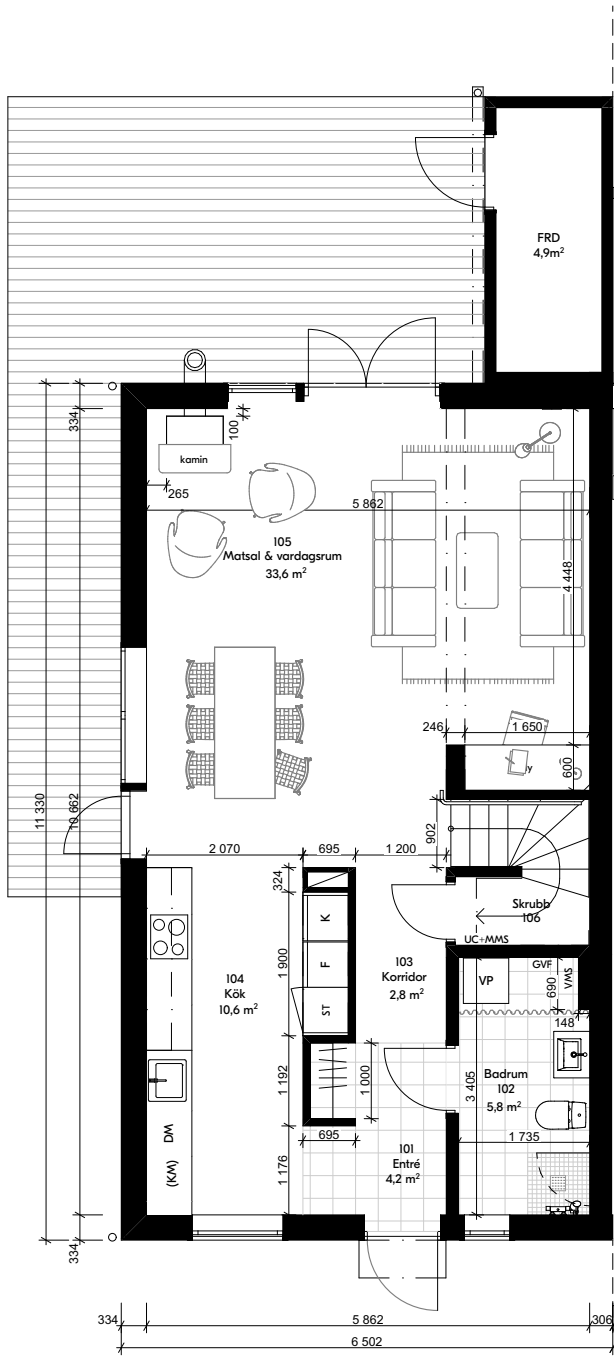
Entréplan
