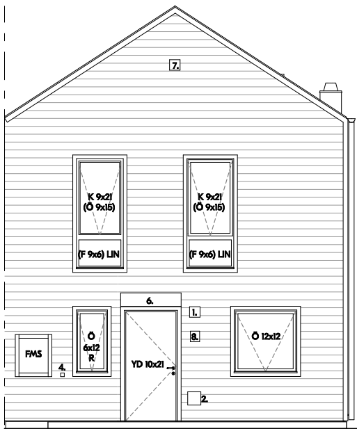
Framsida
