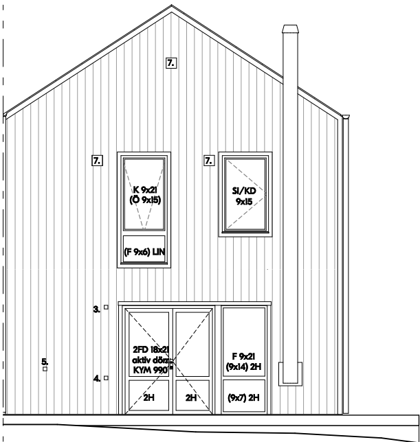
Baksida
