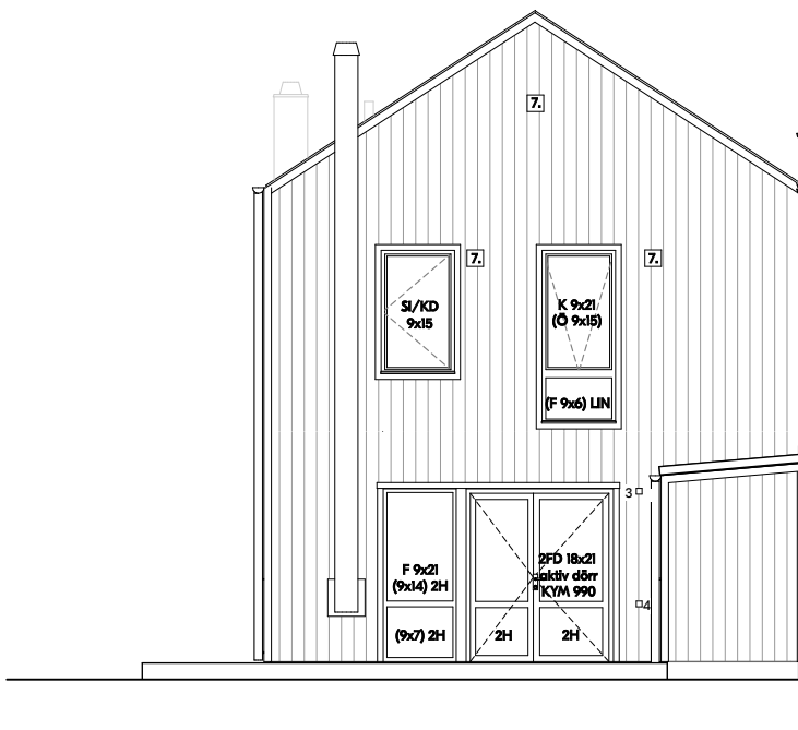
Baksida
