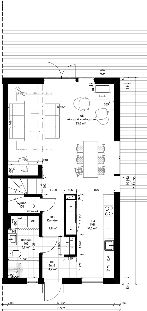
Entréplan
