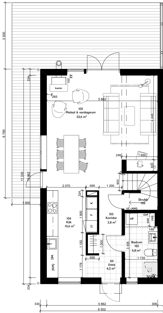
Entréplan
