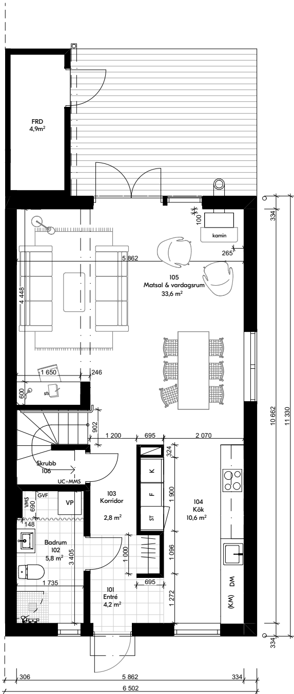
Entréplan
