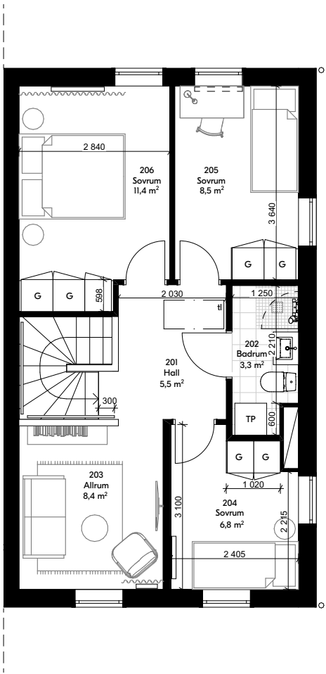
Övre plan
