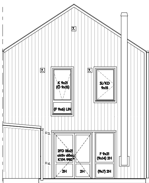
Baksida
