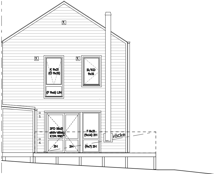
Baksida
