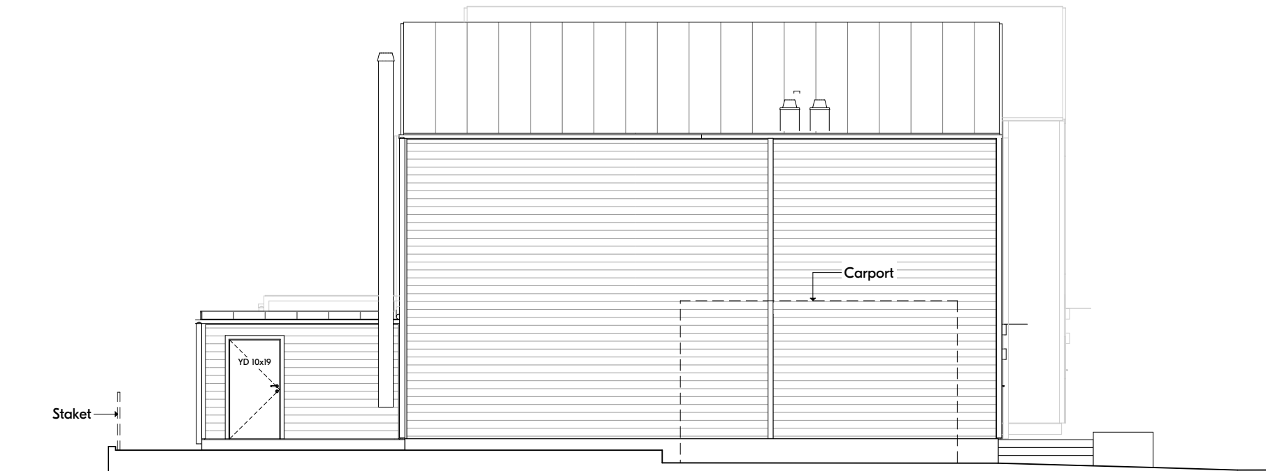
Gavel vänster
