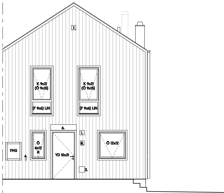
Framsida
