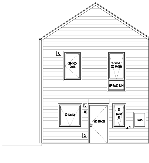
Framsida
