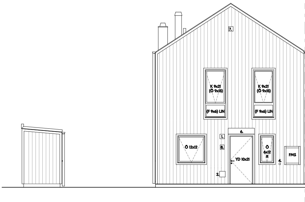
Framsida
