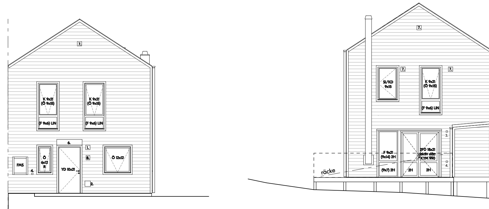
Framsida
