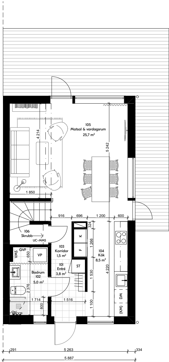
Entréplan
