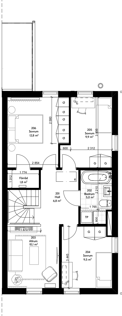
Övre plan
