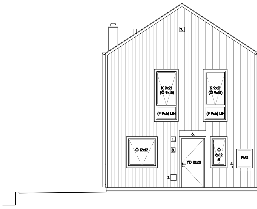
Framsida
