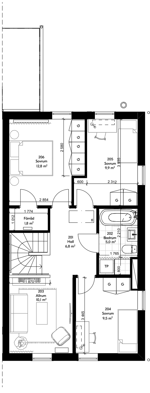
Övre plan
