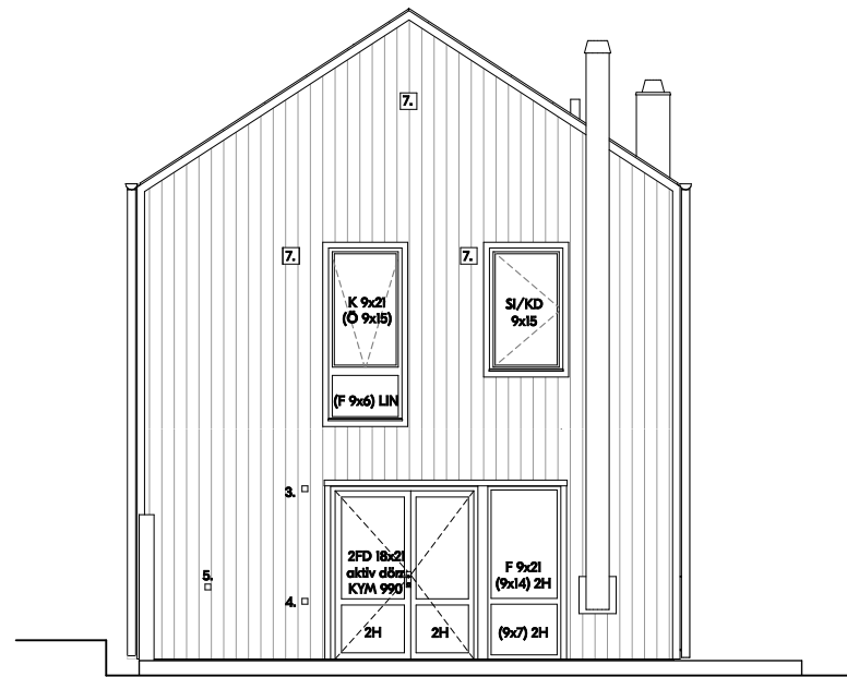
Baksida
