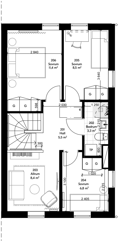
Övre plan
