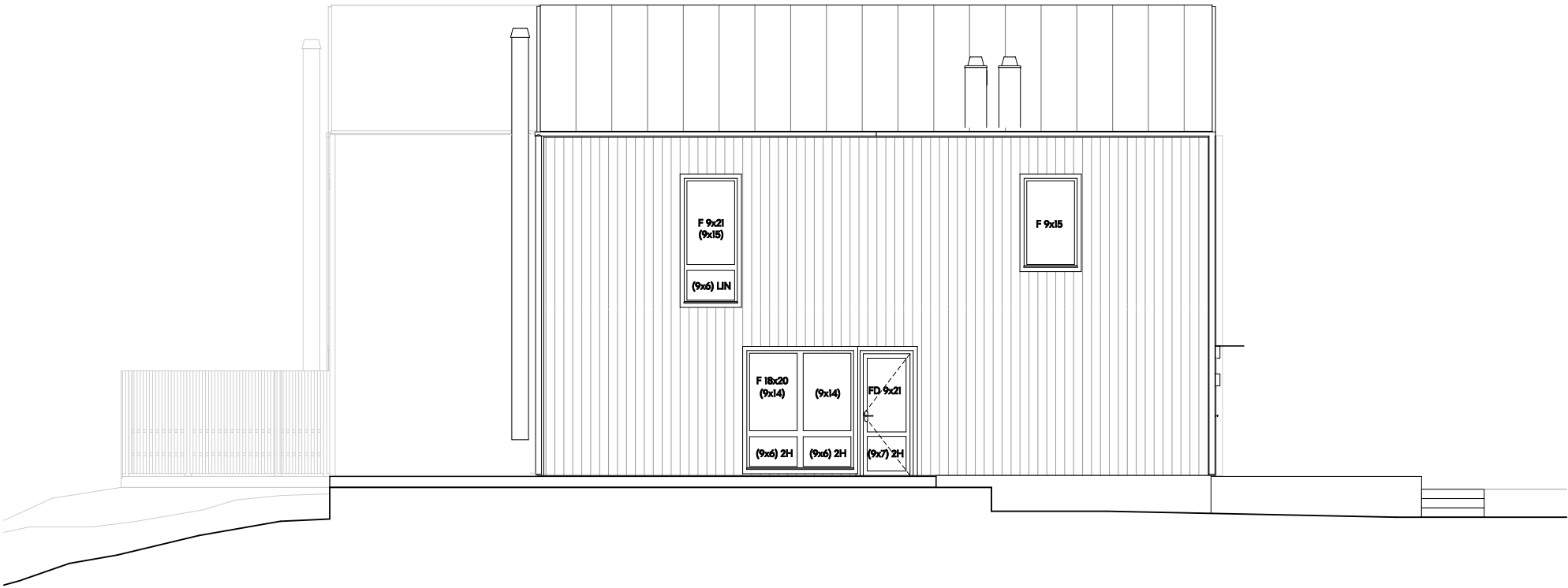
Gavel vänster
