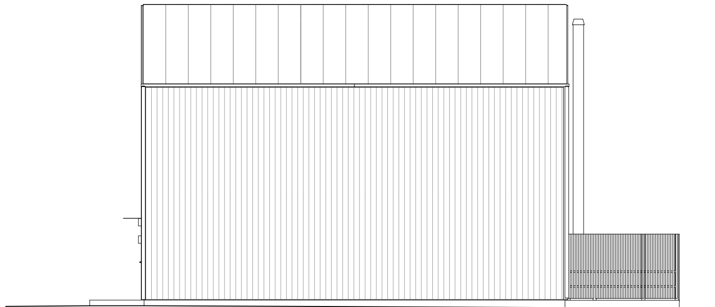
Gavel höger
