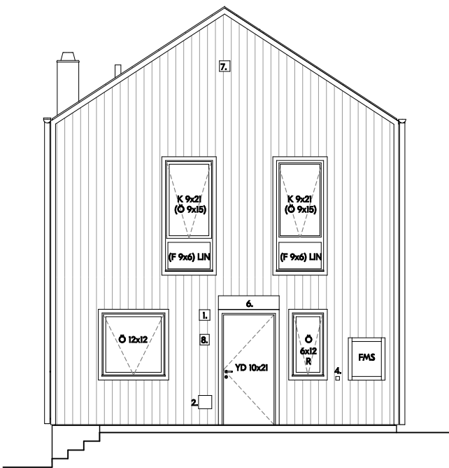
Framsida
