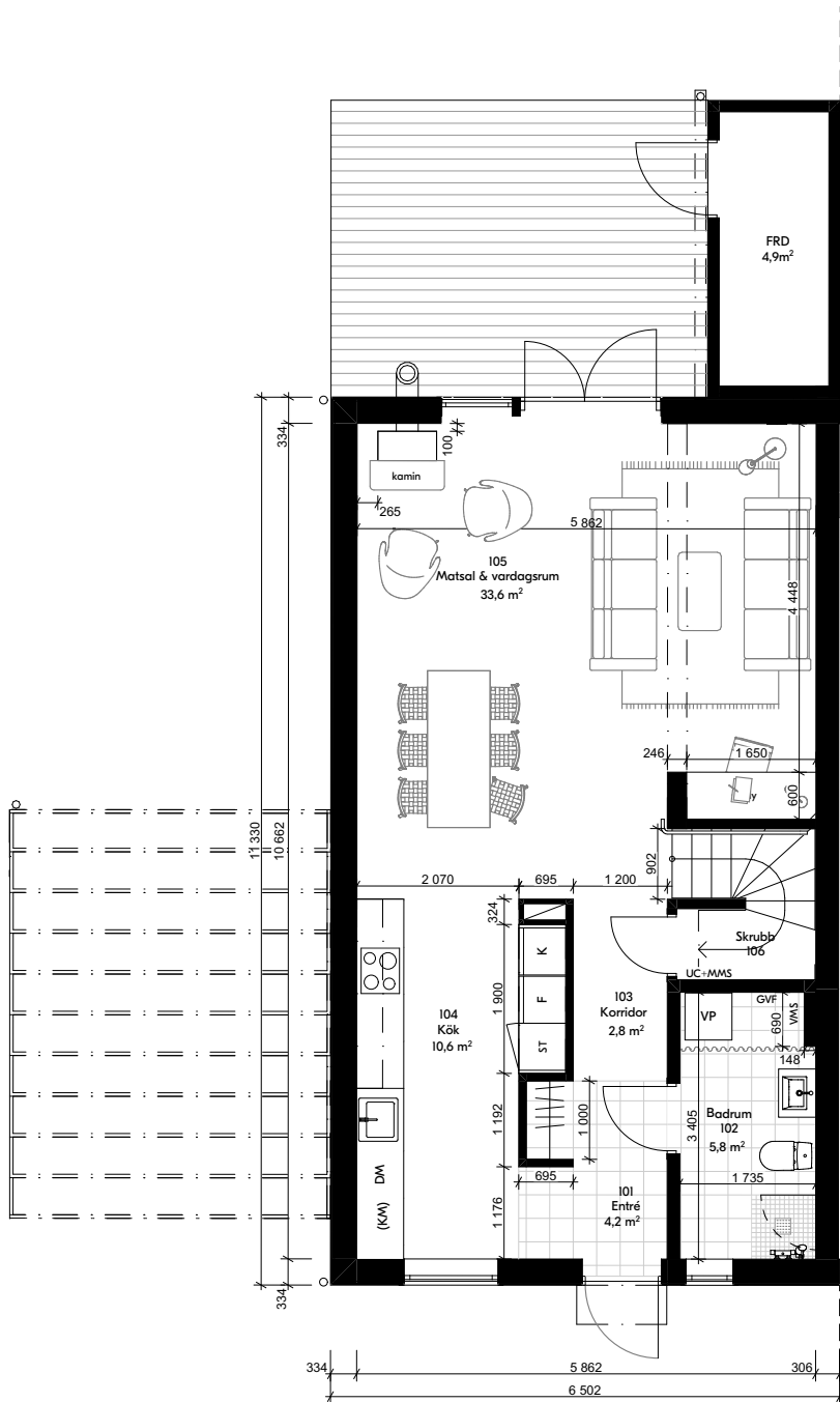
Entréplan
