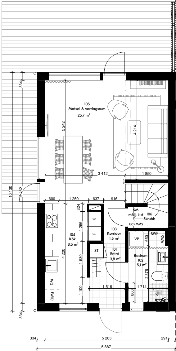
Entréplan
