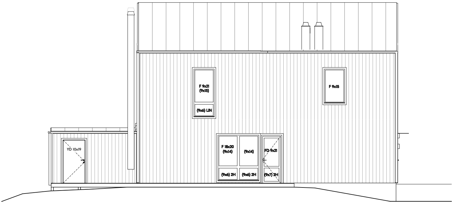
Gavel vänster
