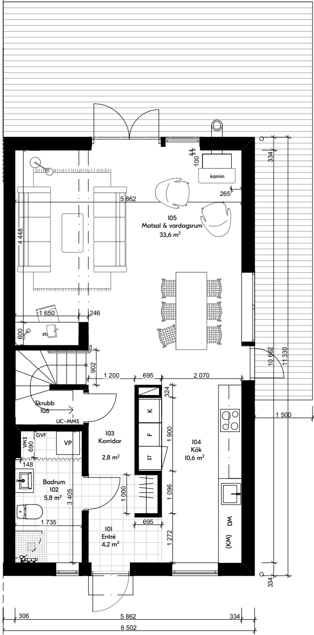
Entréplan
