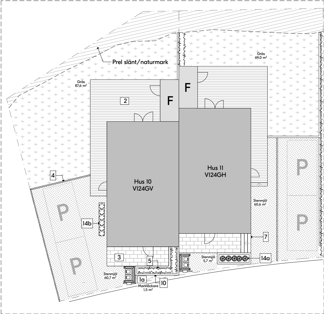
Hus 10-11 Finplanering
