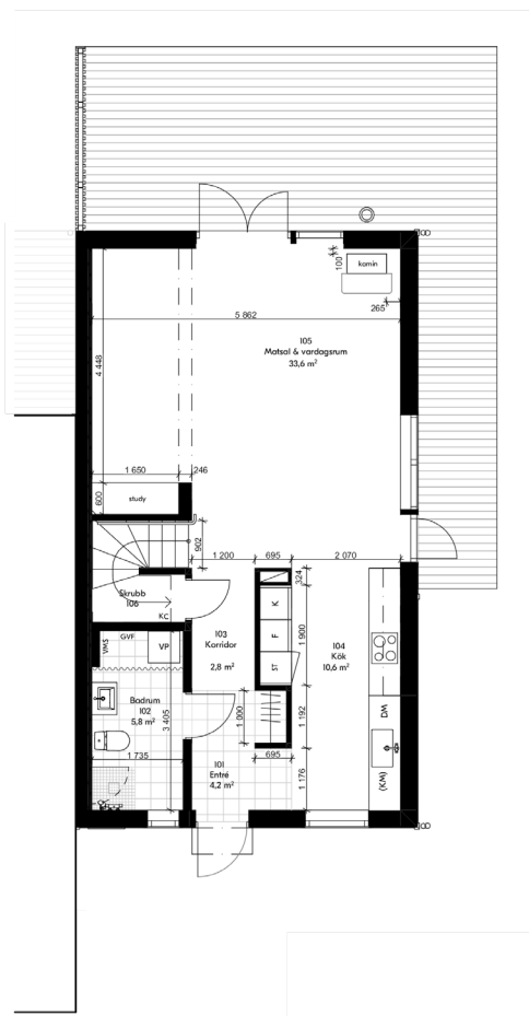
Entréplan
