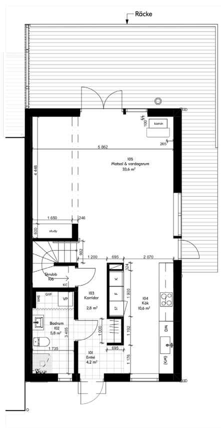
Entréplan
