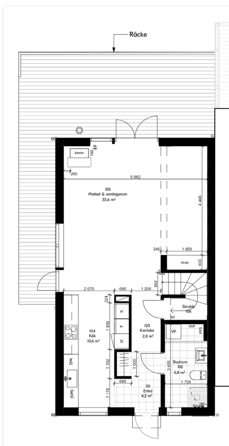
Entréplan
