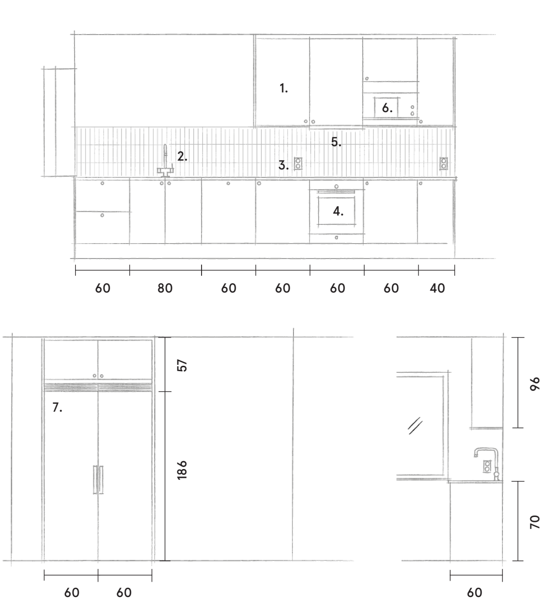
Kök – 99 m 2 (mått angivna i cm)
