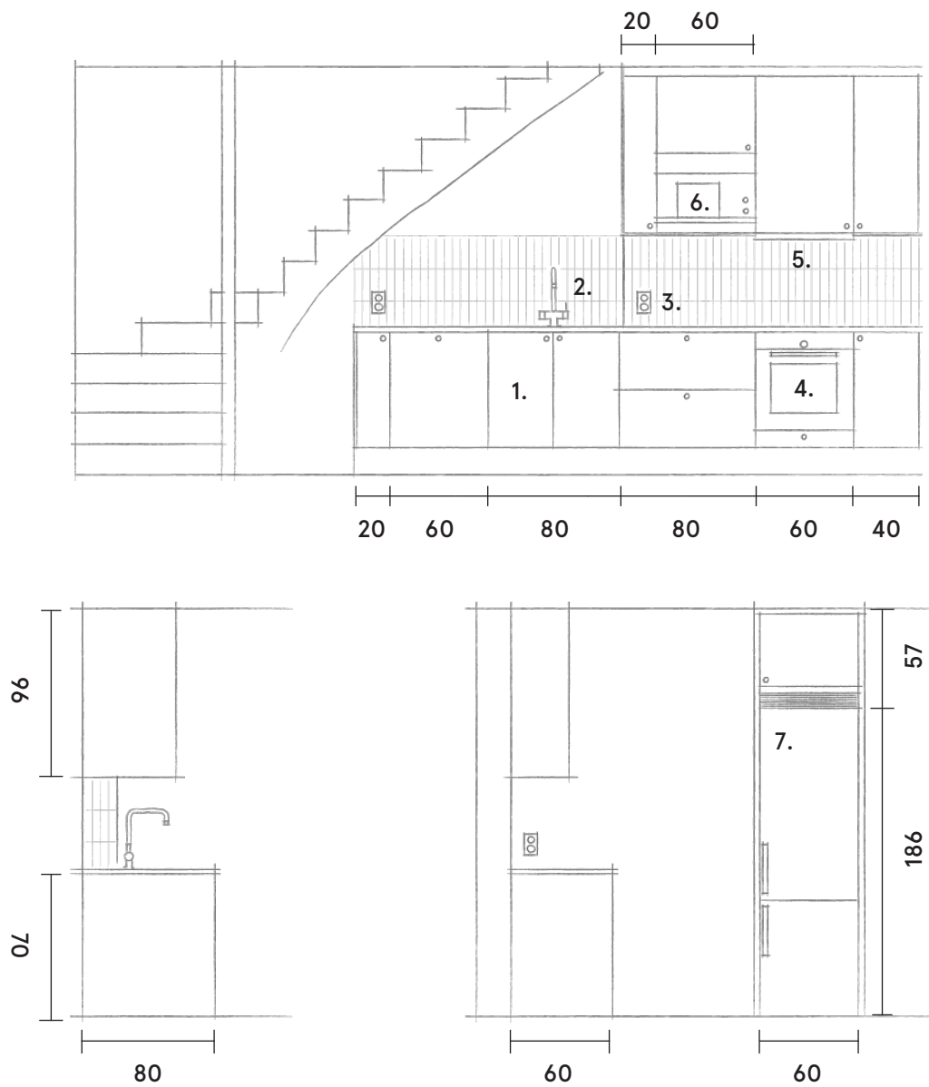
Kök – 73 m 2 (mått angivna i cm)
